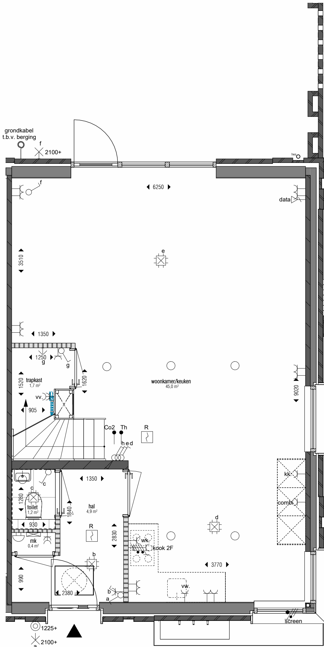
begane grond 1 : 50
