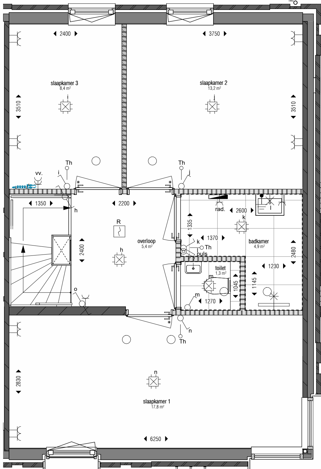
eerste verdieping 1 : 50
