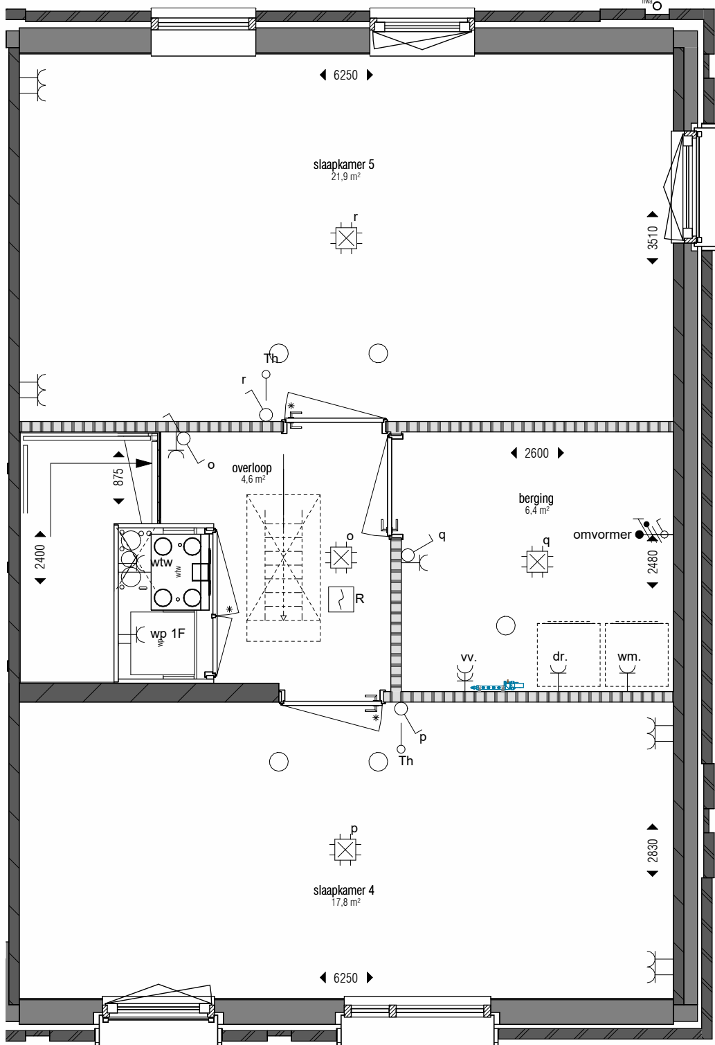
tweede verdieping 1 : 50
