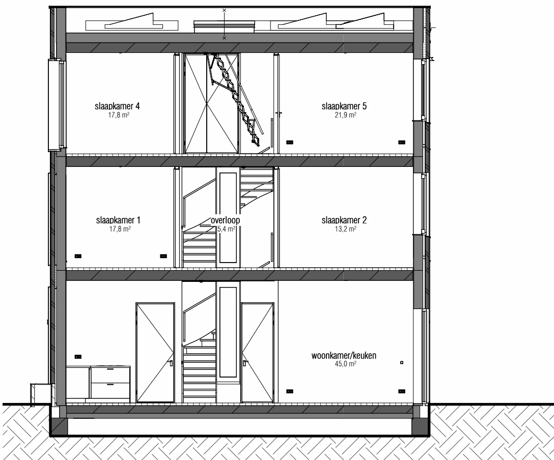
doorsnede 1 : 100
